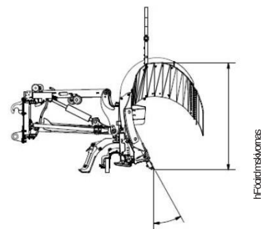
Knivens skärvinkel
